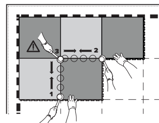
Rys. nr 4 Sposób układania płytek INVISIBLE, BUSINESS
